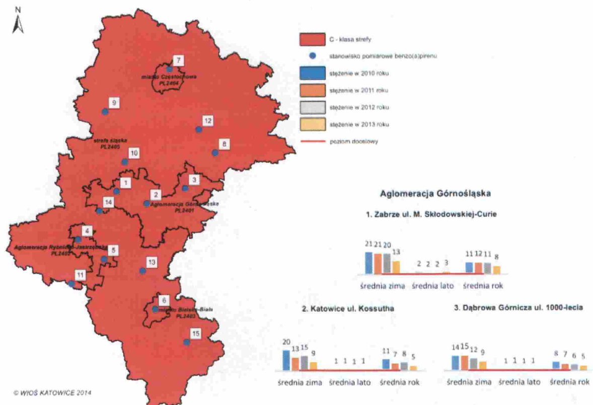
Rysunek 3.1 Wyniki klasyfikacji stref dla benzo(a)pirenu ze względu na ochronę zdrowia ludzi oraz stężenia średnie roczne, w sezonie zimowym i letnim w \text{ng}/\text{m}^3 na stanowiskach pomiarowych w latach 2010-2013 (poziom docelowy 1 \text{ ng}/\text{m}^3 )
