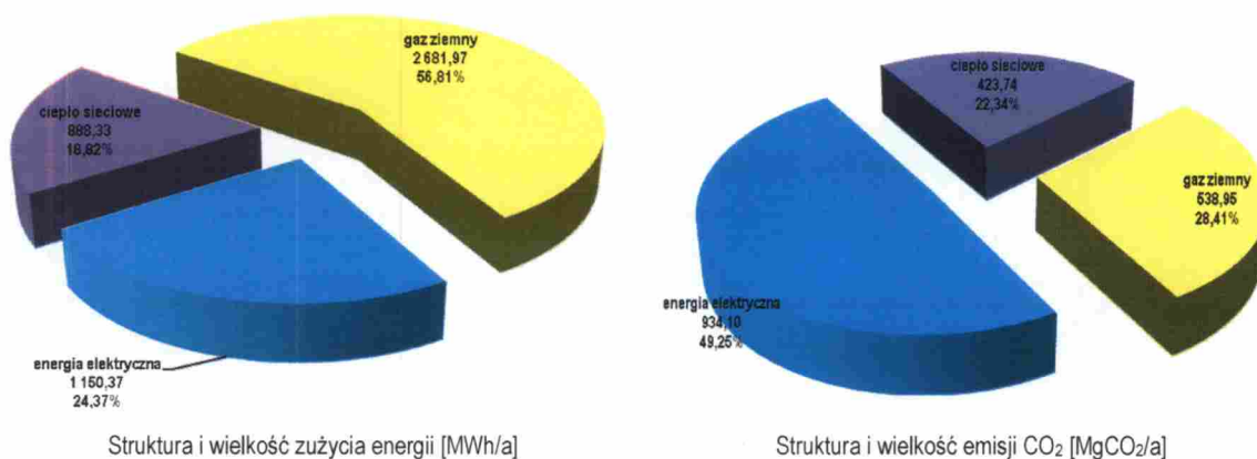
Wykres 5.3. Struktura zużycia energii oraz emisji CO 2 – pozostałe obiekty/instalacje komunalne (rok bazowy)
