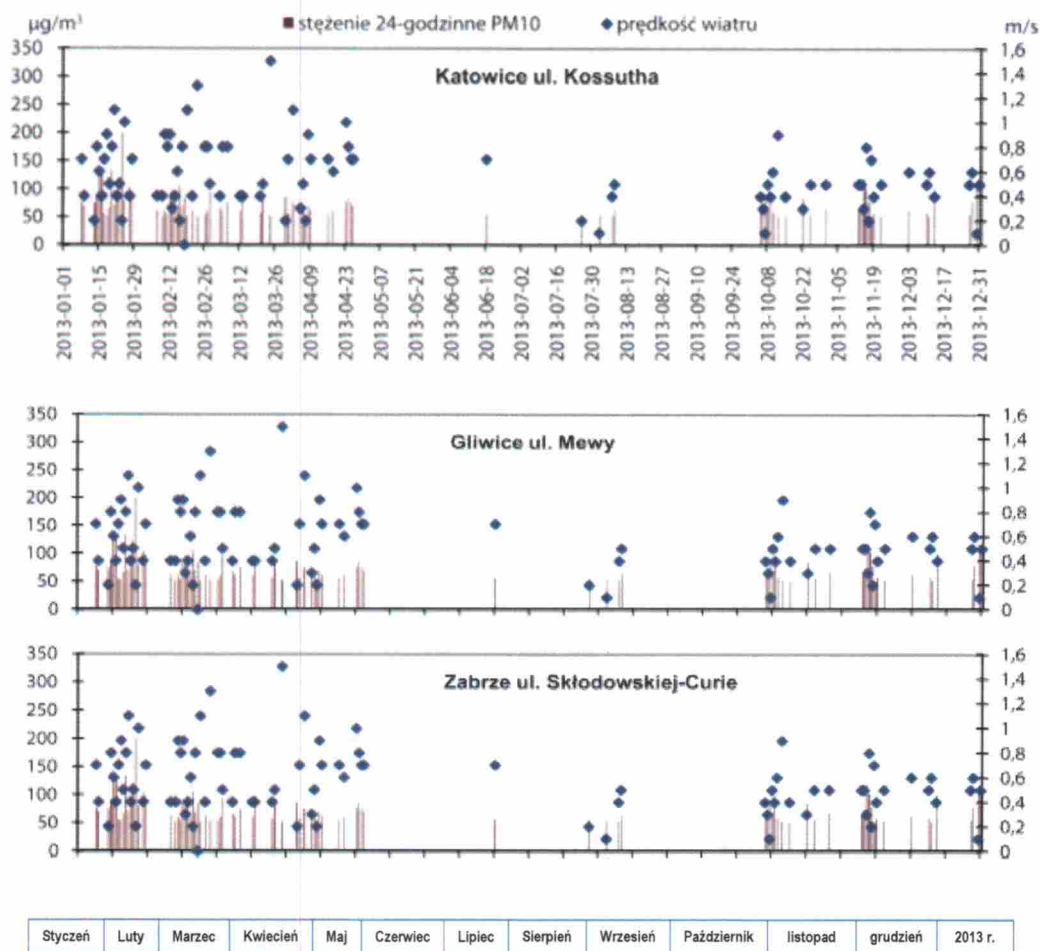
Wykres 3.2. Rozkłady prędkości wiatru poniżej 1,5 m/s oraz 24-godzinnych stężeń pyłu zawieszonego PM10 przekraczające poziom dopuszczalny 50 \mu\text{g}/\text{m}^3 w aglomeracji górnośląskiej w 2013 roku
