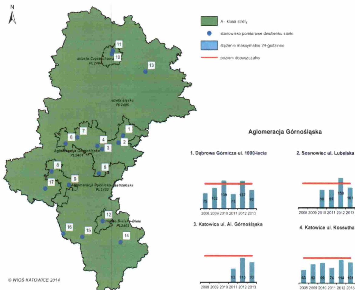
Rysunek 3.2 Wyniki maksymalnych stężeń 24-godzinnych dwutlenku siarki w \mu\text{g}/\text{m}^3 na stanowiskach pomiarowych w latach 2008-2013 oraz klasyfikacja stref w 2013 roku ze względu na ochronę zdrowia ludzi (poziom dopuszczalny dla stężeń 24-godzinnych - 125 \mu\text{g}/\text{m}^3 )
