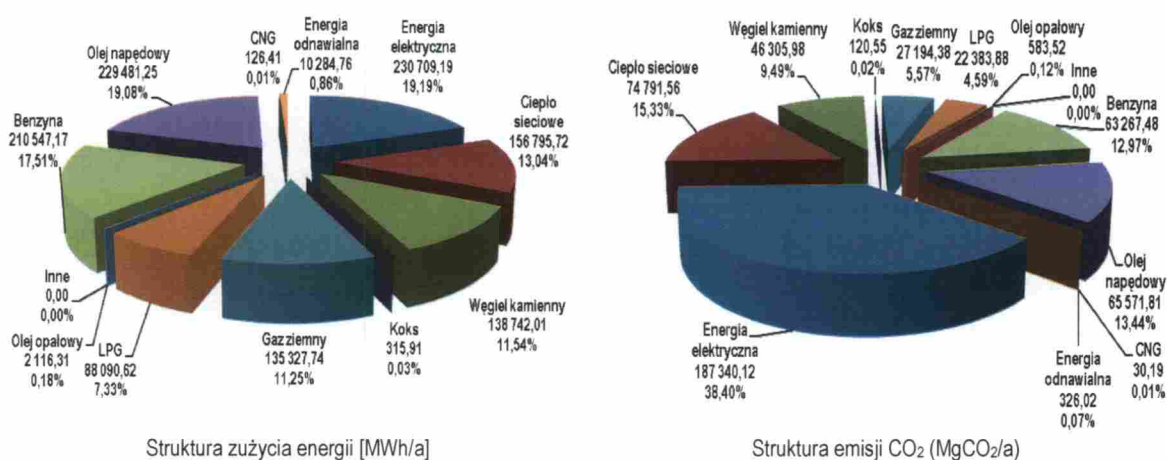
Wykres 5.8. Struktura zużycia energii i emisja CO 2 – ujęcie graficzne
